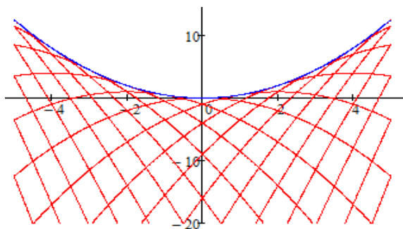
Интегральные кривые уравнения (278.1) (парабола 2y = x^2 – огибающая семейства парабол 4y = C^2 - 2(x - C)^2 )
