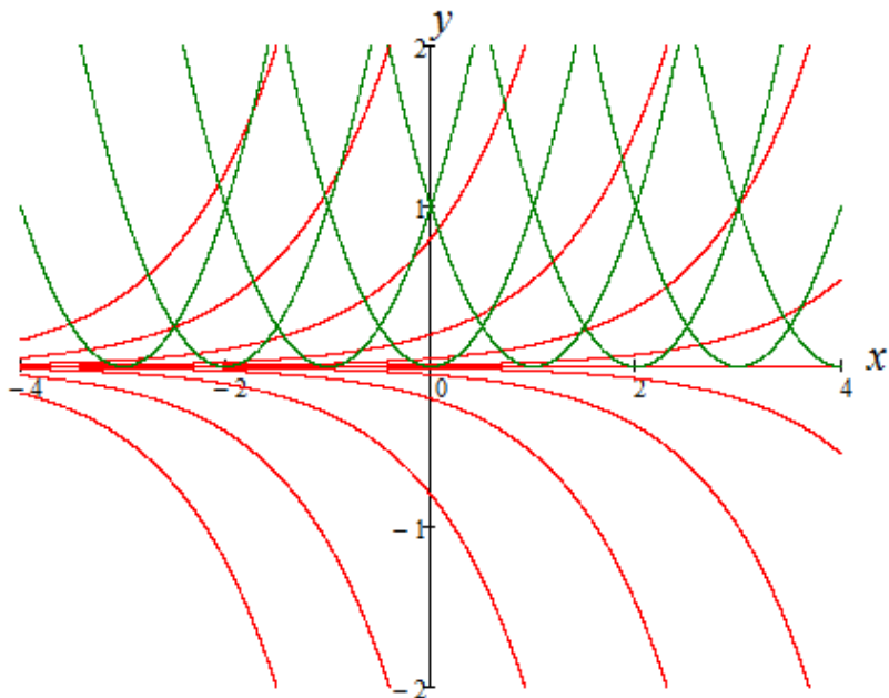
Рис. 4. Интегральные кривые уравнения (249.1)
